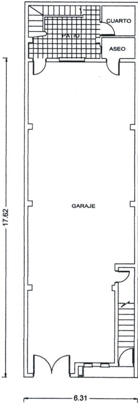
PLANTA BAJA
