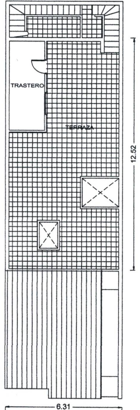
PLANTA CUBIERTA
